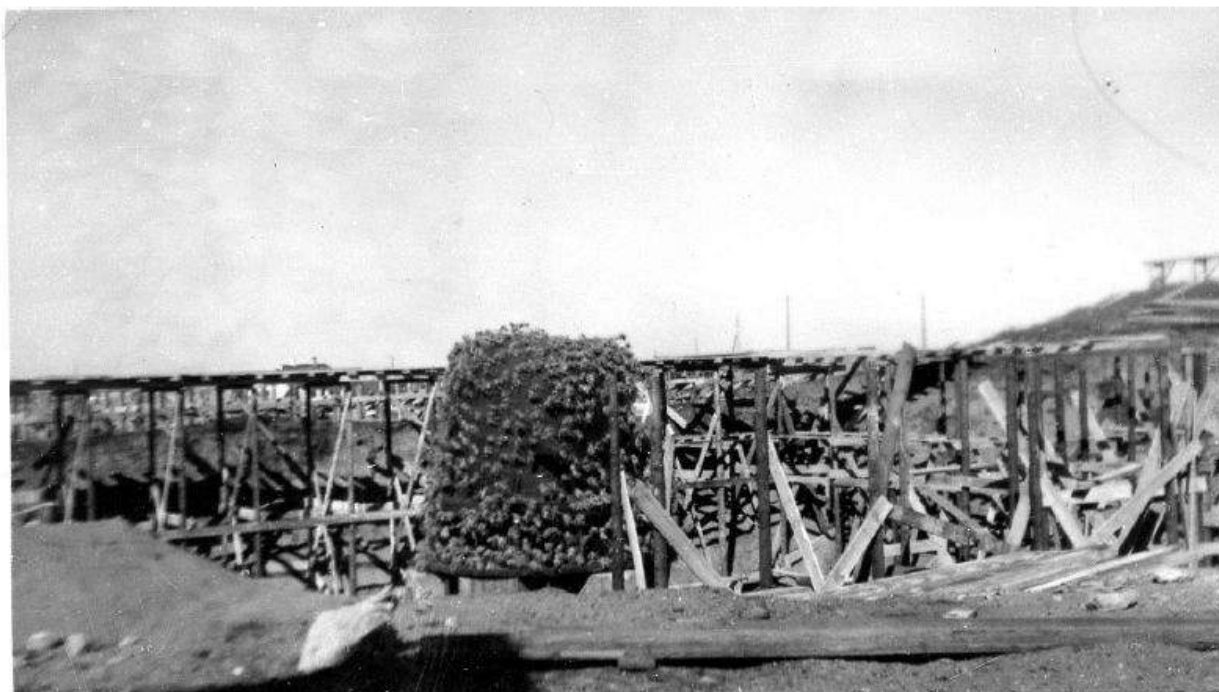
Hullet til bunkeren er færdiggravet, og som noget af det første er panserkuplen til mortéren blev placeret på betonpiller på støbesålen. Træstilladset tjente formentlig som tilkørselsrampe for betonen til støbningen af pilleme under kuplen. (4968)
